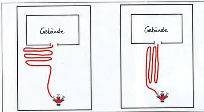
Verlegerichtung: Die ausgelegte Schlauchreserve quer zur Treppe hat sich als unvorteilhaft erwiesen, da sie um eine Ecke und die Treppe hinauf führt. Die Schlauchkupplungen bleiben am Geländer und den Treppenstufen hängen, damit ist die Arbeit der Atemschutztrupps im Gebäude erschwert.
